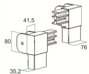
Esquinero triple
