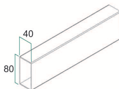
Perfil 80x40
